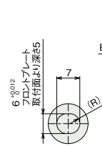
詳細図 P ベース長穴/テーブル長穴詳細 詳細図 Q フロントプレート長穴詳細
