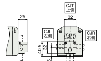
ケーブル取出方向 (オプション)
