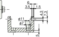
断面図 Z-Z Tスロットとベース取り付け用座ぐり穴詳細
