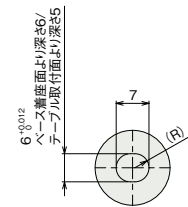
詳細図 P ベース長穴/テーブル長穴詳細 詳細図 Q フロントプレート長穴詳細
