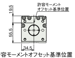
許容モーメントオフセット基準位置
