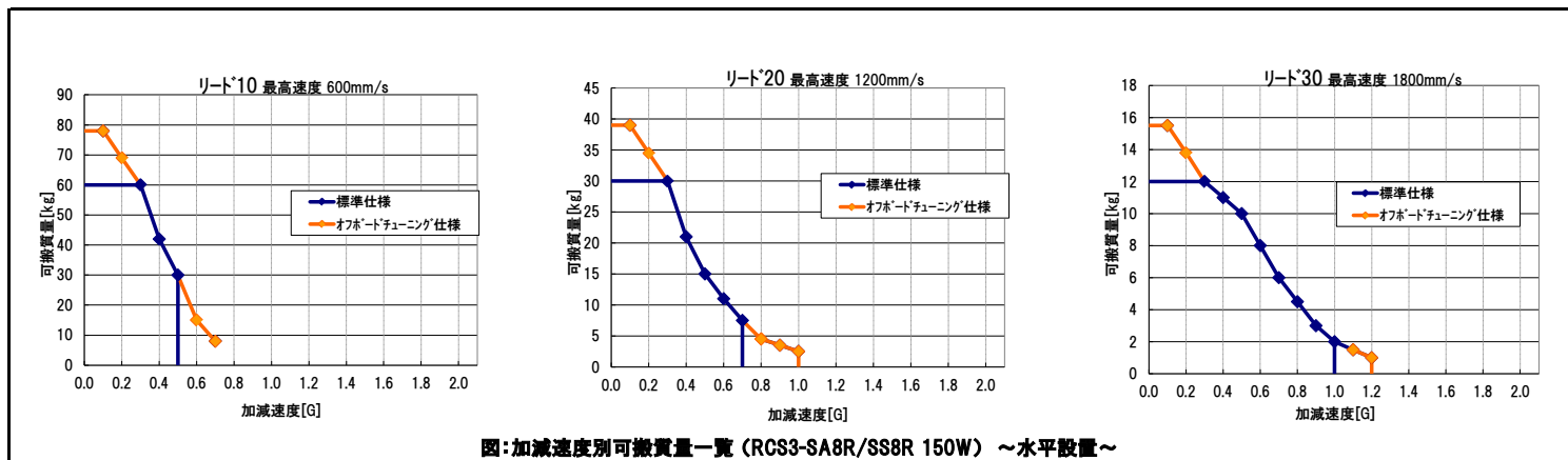
図:加減速度別可搬質量一覧 (RCS3-SA8R/SS8R 150W) ~水平設置~
