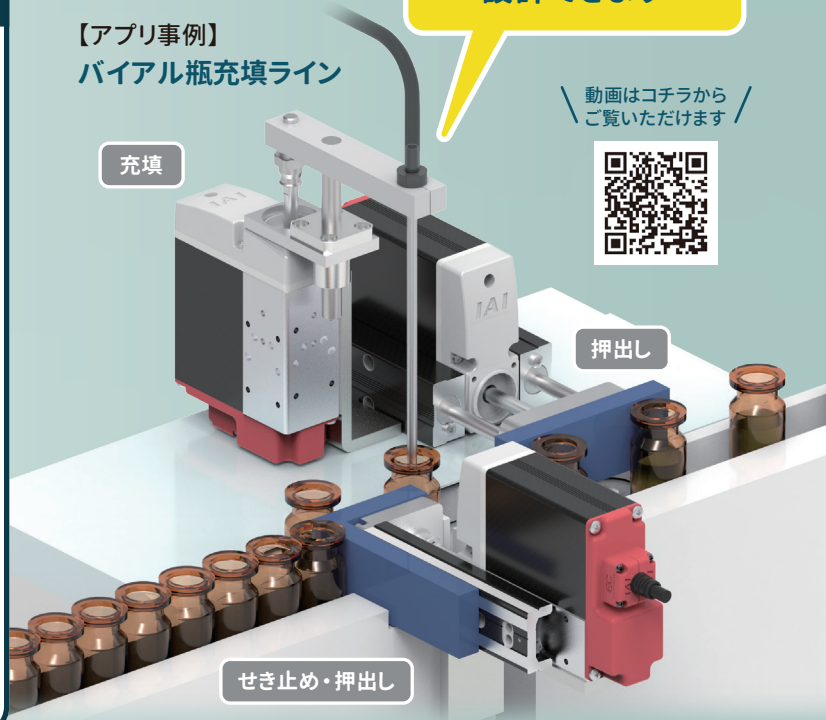
ダブルガイド付きロッド (GD3)
