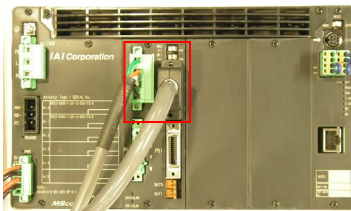
制御電源入力コネクタ正面図
