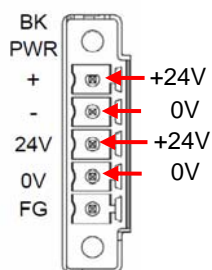
制御電源入力コネクタ正面図
